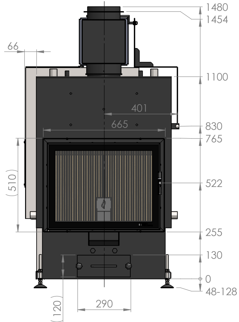
WYMIARY - LOUIS AQUA 15kW ZE ZBIORNIKIEM 30 kg
