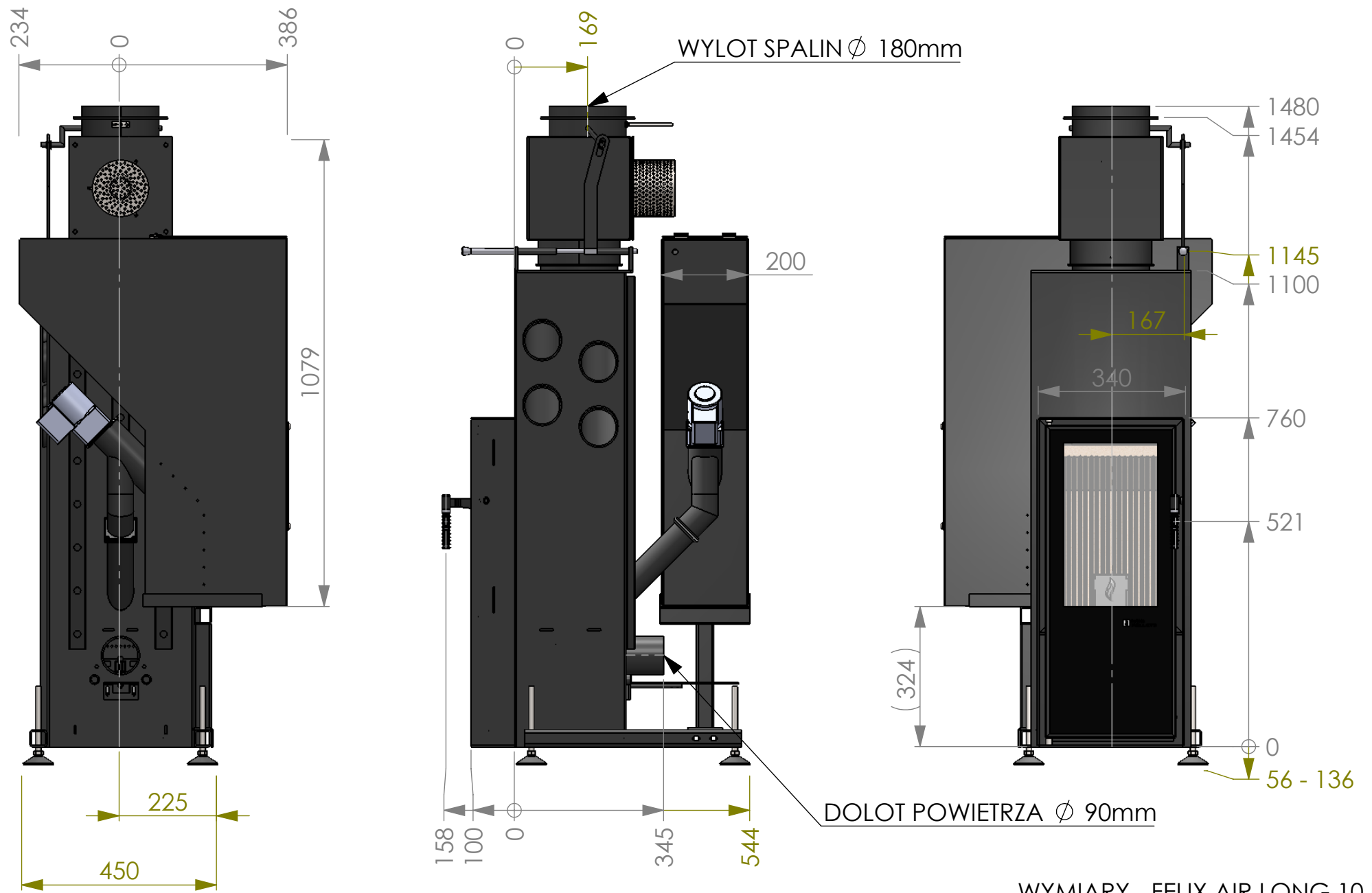
WYMIARY - FELIX AIR LONG 10 kW
